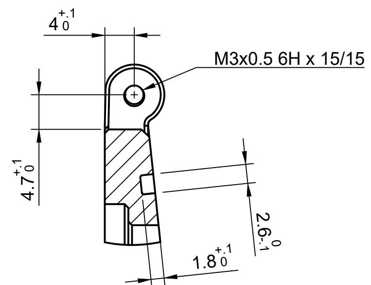
C (2:1)
