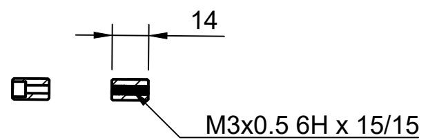
A-A (1:2)
